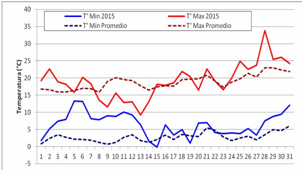
Gráfico 3. Línea de puntos: promedio histórico de temperaturas máximas y mínimas diarias de agosto. Línea continua: temperaturas máximas y mínimas diarias registradas durante el mes de agosto de 2015.
